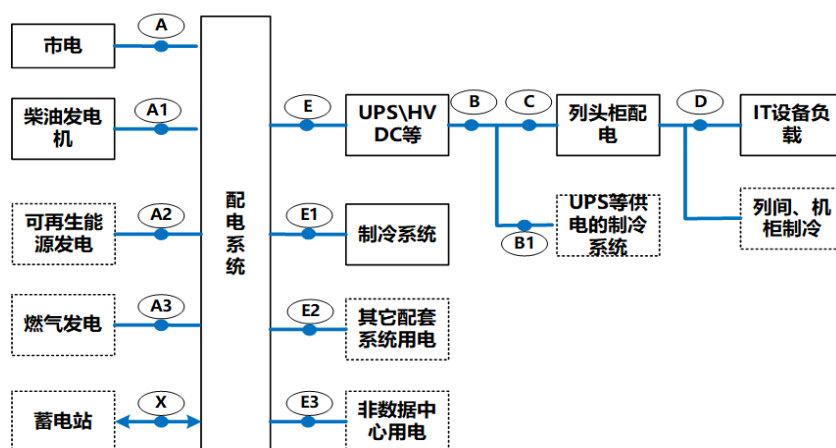
图 A.1 数据中心电能消耗测量点示意图
