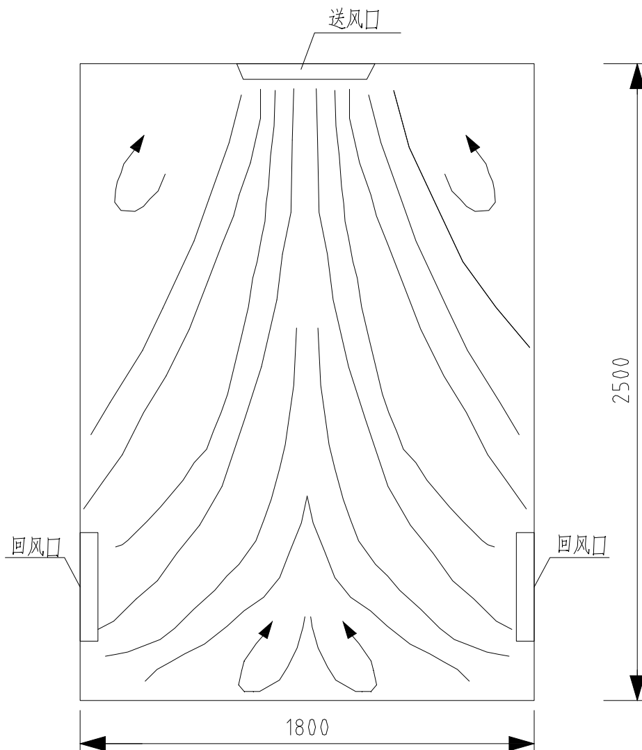
图 2 气流组织形式下室内流场分布
