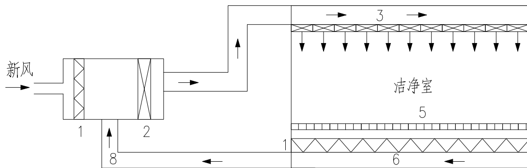
图1 垂直单向流洁净室原理图
